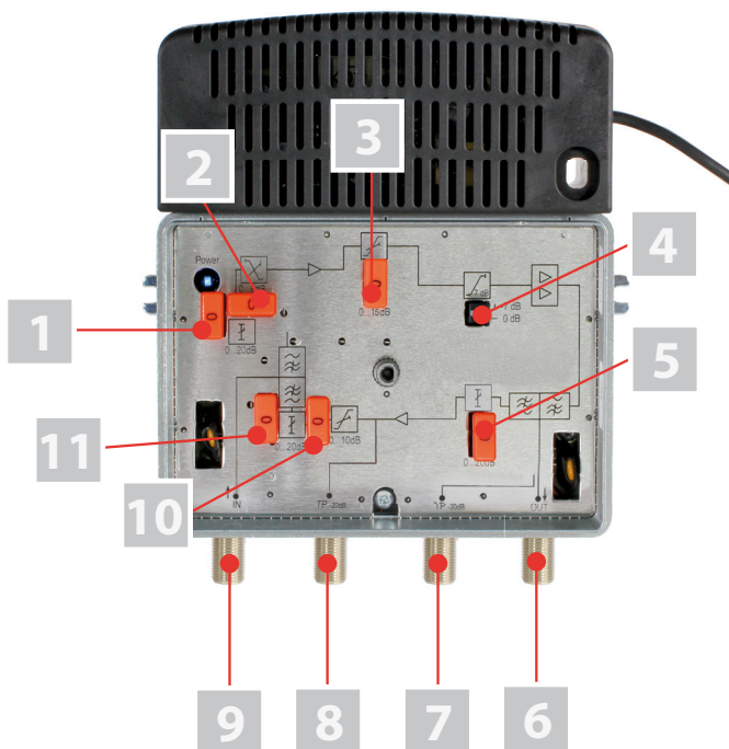
Bild 2: Verstärker HV 536, Innenansicht
